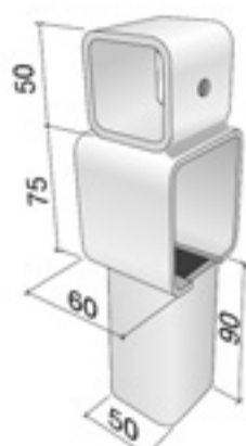
Ändstopp dubbelkonsol
