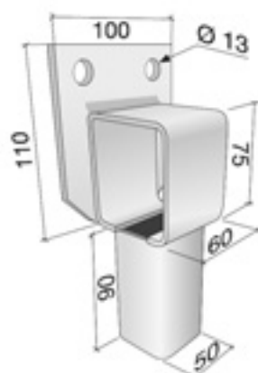
Ändstopp enkelkonsol
