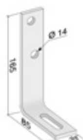
Fästjärn enkelt
