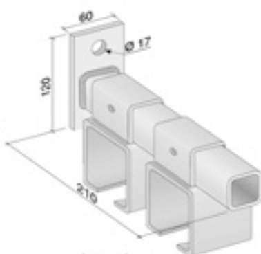
Justerbar dubbelkonsol
